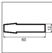
TUBULÁRNÁ LAMELA TUBULÁRNÍ LAMELA
