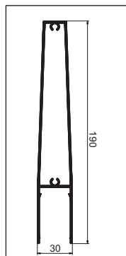
DEKORATIVNÁ LAMELA DEKORATIVNÍ LAMELA
