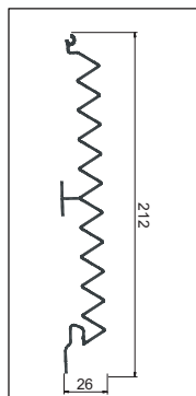
TVAROVANÁ LAMELA TVAROVANÁ LAMELA
