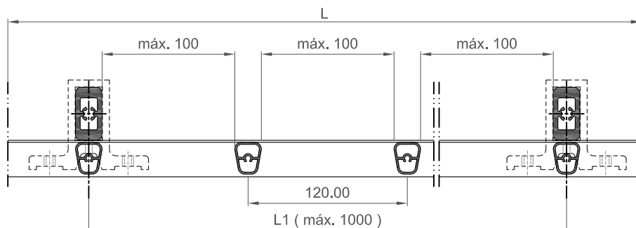
SECCIÓN A-A
