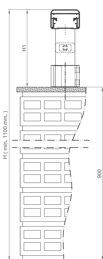
SECCIÓN B-B
