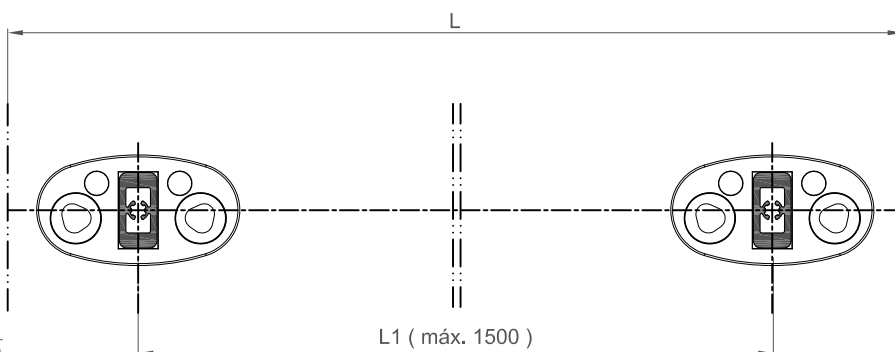
SECCIÓN A-A
