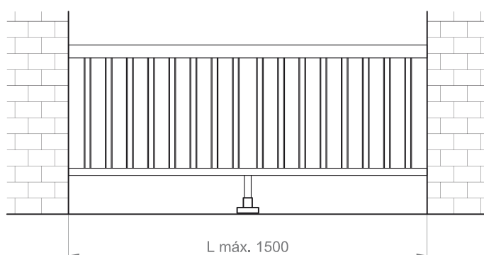
BARANDA ANCLADA AL FRENTE DE FORJADO
