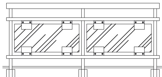
BARANDA ANCLADA AL FRENTE DE FORJADO
