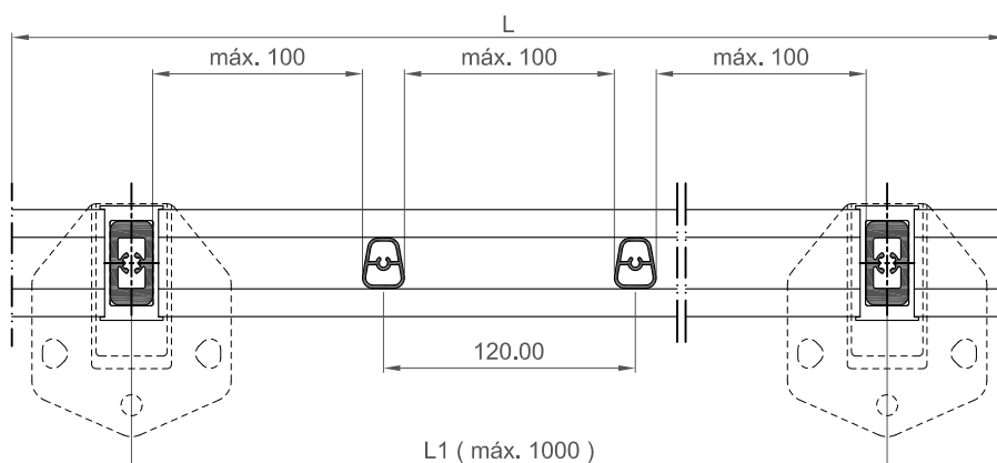
SECCIÓN A-A
